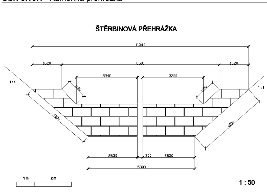
Obr. 8.10.2 Štěrbínová přehrážka
