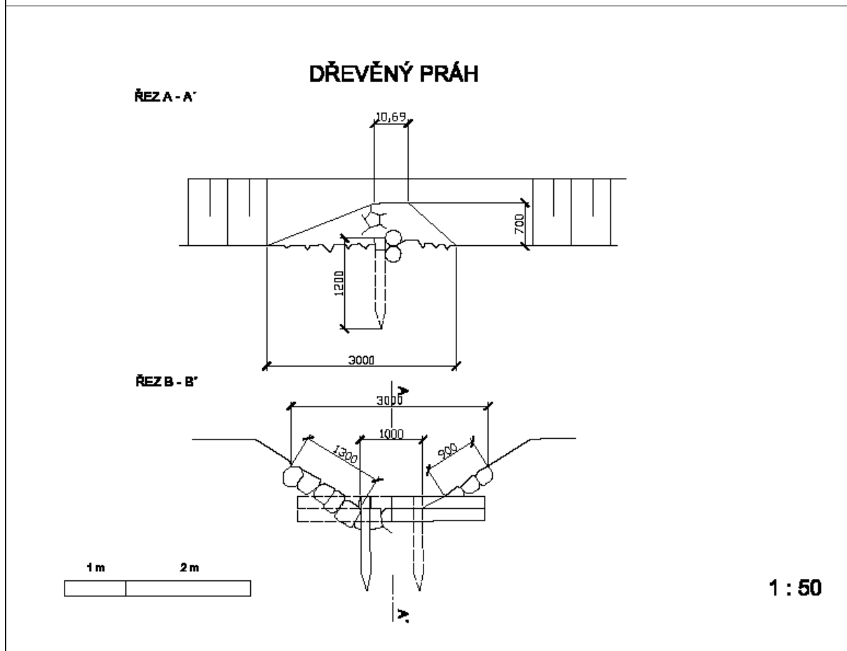
Obr.8.4.1 Dřevěný práh ve dně.
